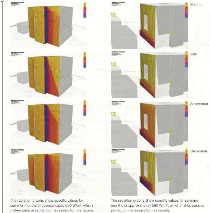
Figura 4. Diagrama del Media-TIC. El nivel de radiación que recibe el edificio en verano es muy elevado, debido al clima de Barcelona.
